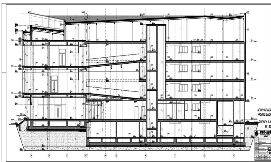
Попречни пресек зграде
